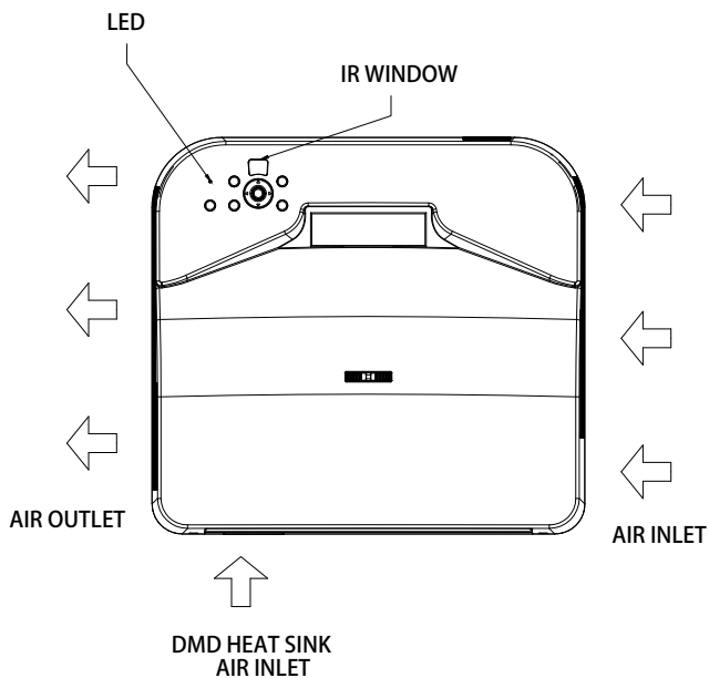
风道走向示意图
